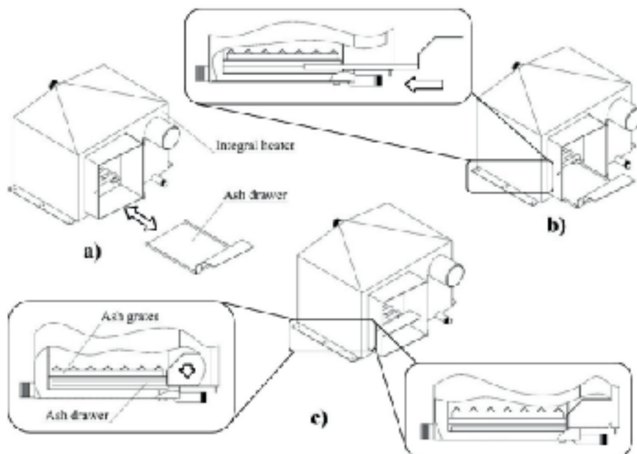
Abbildung 5 Platzierung des Aschefachs (Montageschritt 6).
